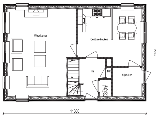
Begane grond alternatief 2
