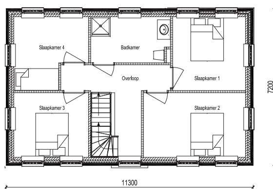
Verdieping alternatief 2
