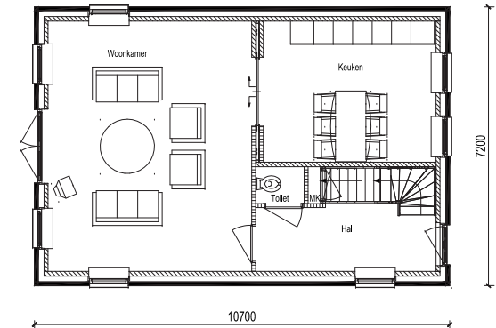
Begane grond alternatief 3
