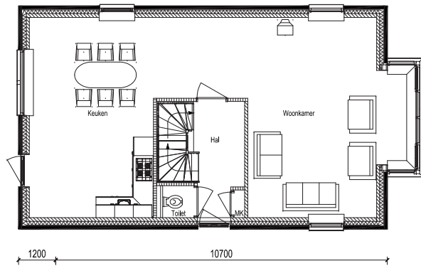
Begane grond alternatief 1
