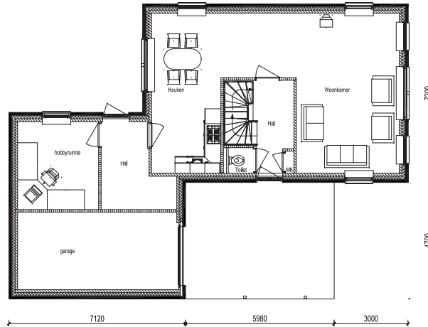
Begane grond alternatief 2
